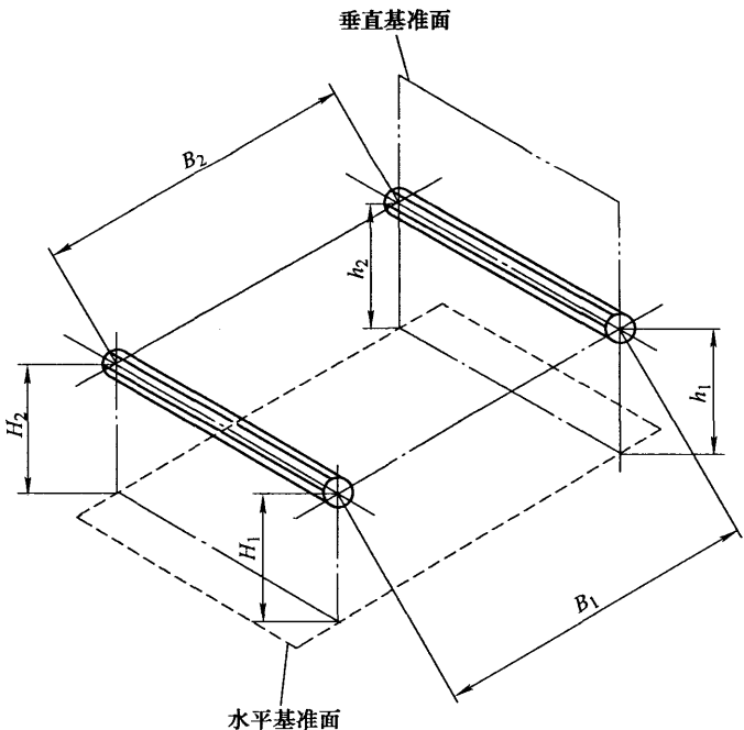
图 1 双轴安装平行度测量
