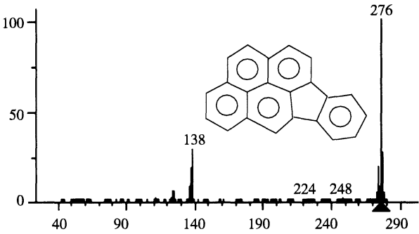
茚并[1,2,3-cd]芘
