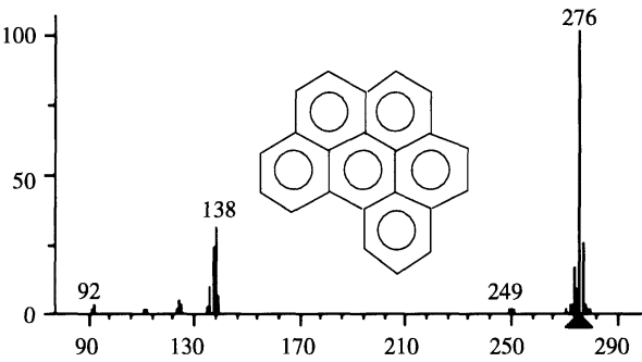
苯并[ghi]花
