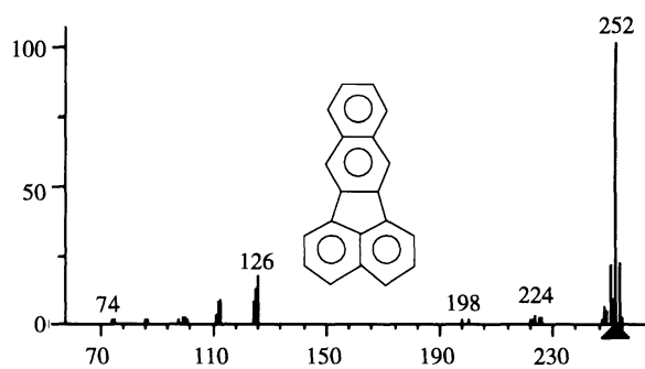
苯并[k]蒽
