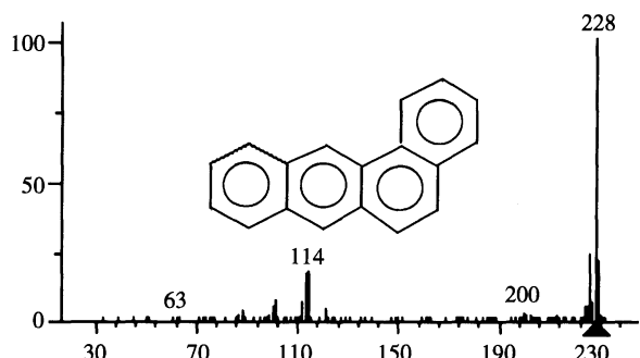
苯并[a]蒽
