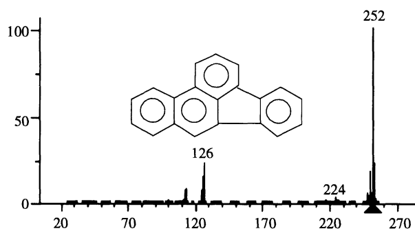
苯并[b]蒽
